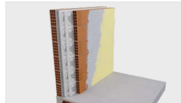
PARETE IN LATERIZIO CON INTERCAPEDINE
