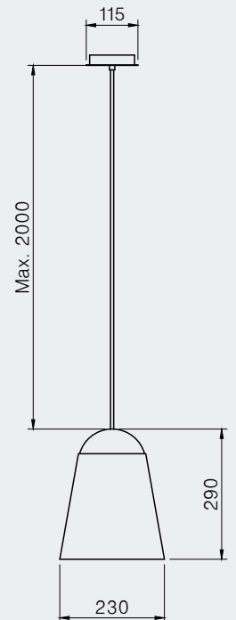
ALB41 IP20 E27 GLS60 led 10w 2700K 810lm
